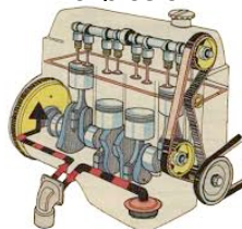
Moteur à explosion
